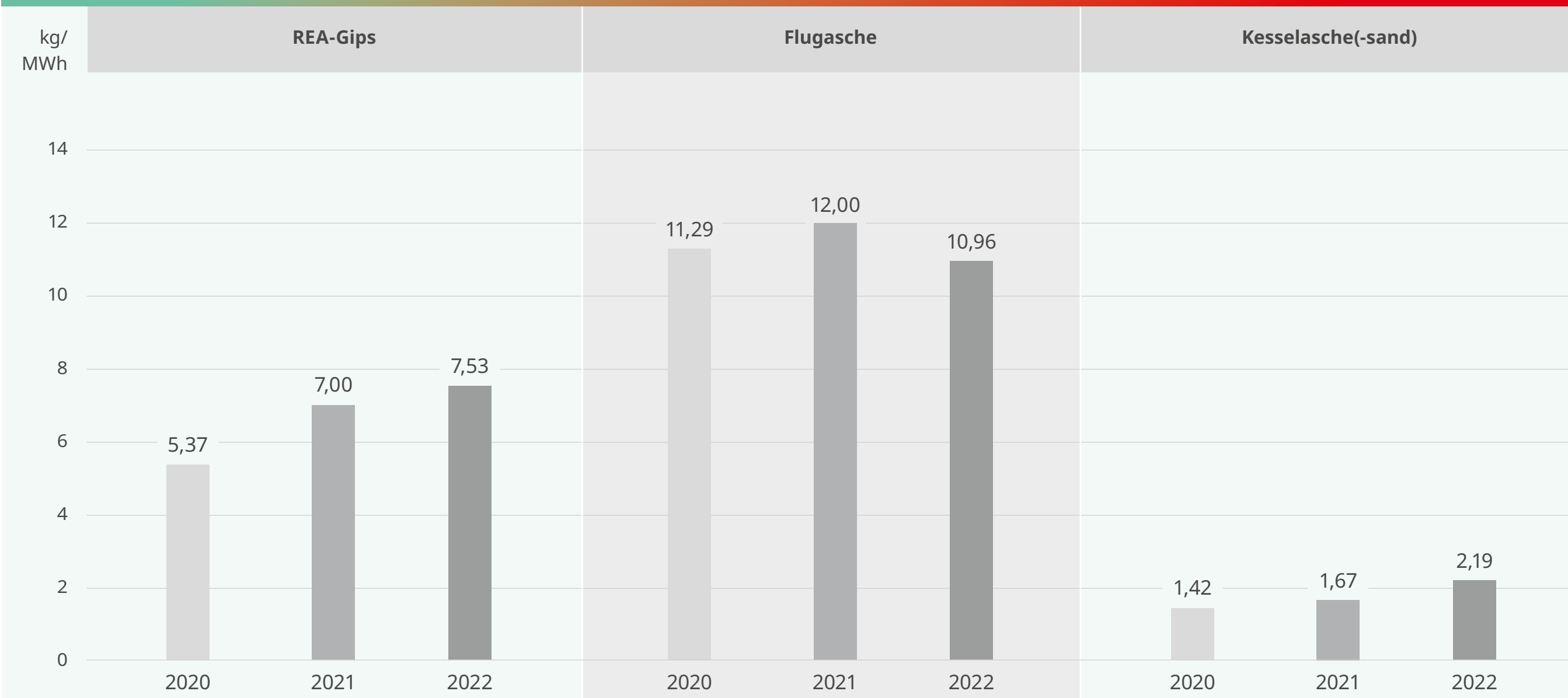
Abbildung 15 Spezifische Nebenprodukte Erzeugung in Block 15 (Heizkraftwerk Hastedt) 2020–2022
