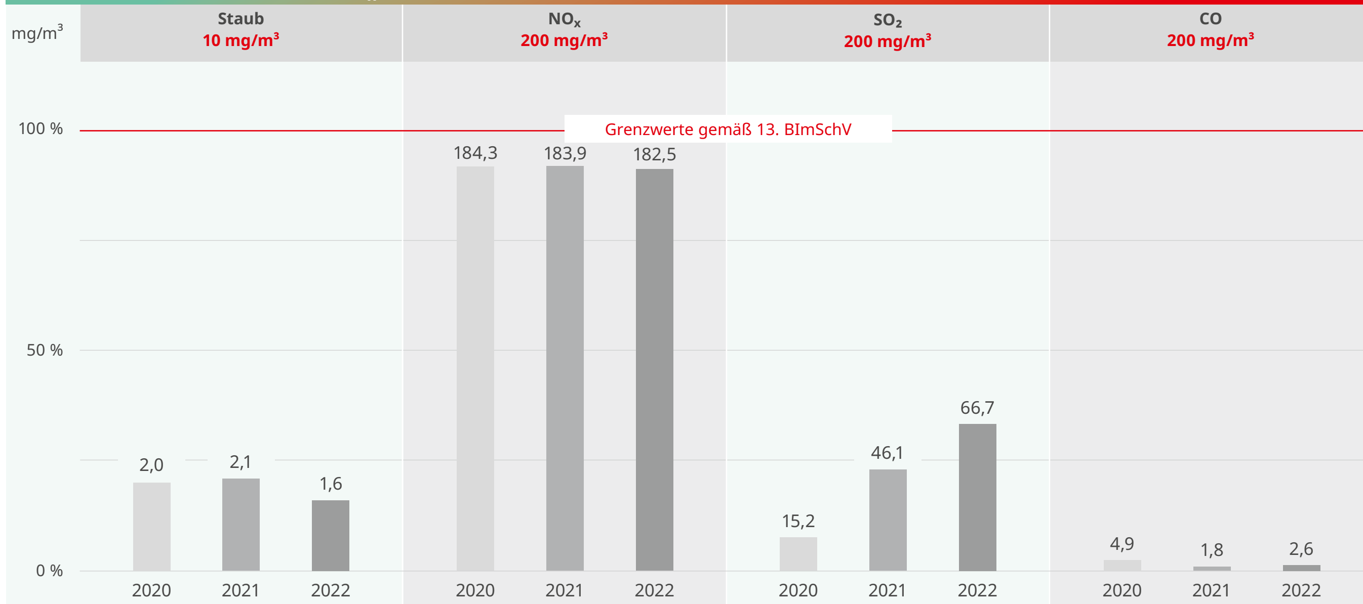
Abbildung 5 Emissionen Staub, NO x , SO 2 und CO (in mg/m 3 ) Heizkraftwerk Hastedt (Block 15) 2020–2022
