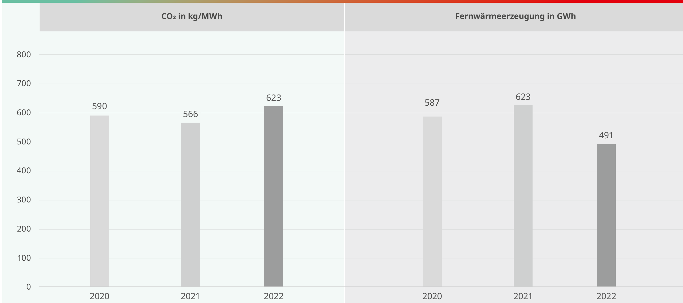
Abbildung 17 Spezifische CO 2 -Emissionen und Fernwärmeerzeugung (swb Erzeugung) 2020–2022
