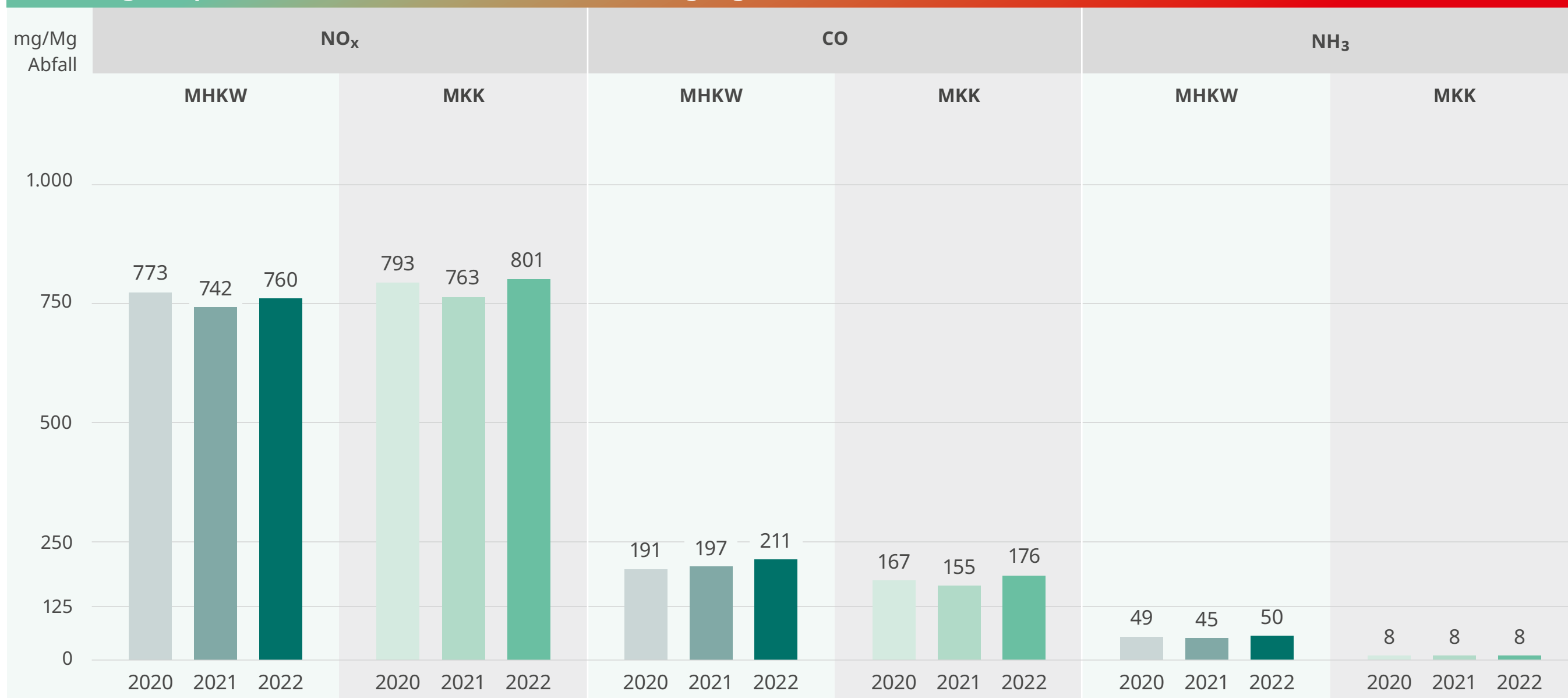
Abbildung 12 Spezifische Frachten NO x , CO und NH 3 (in mg/Mg) MHKW und MKK 2020–2022
