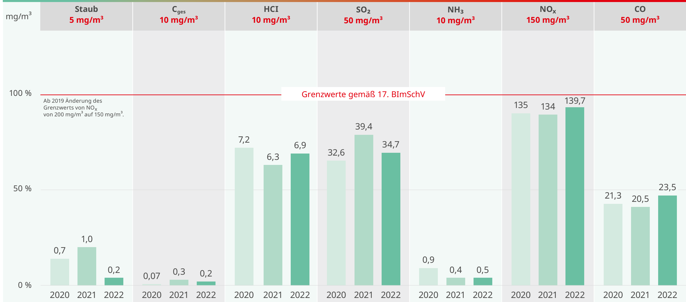
Abbildung 8 Vergleich der kontinuierlich gemessenen Emissionen (in mg/m 3 ) MKK 2020–2022
