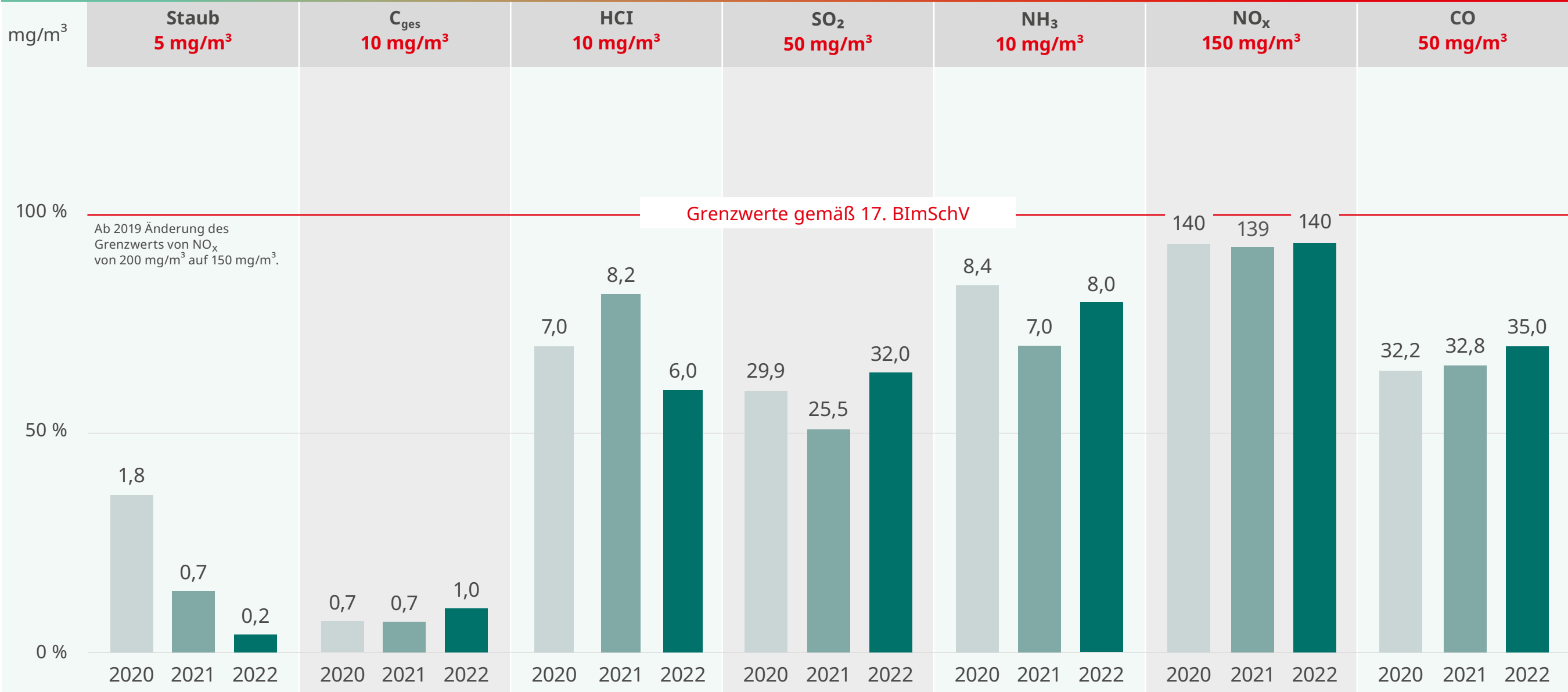
Abbildung 7 Vergleich der kontinuierlich gemessenen Emissionen (in mg/m 3 ) MHKW 2020–2022
