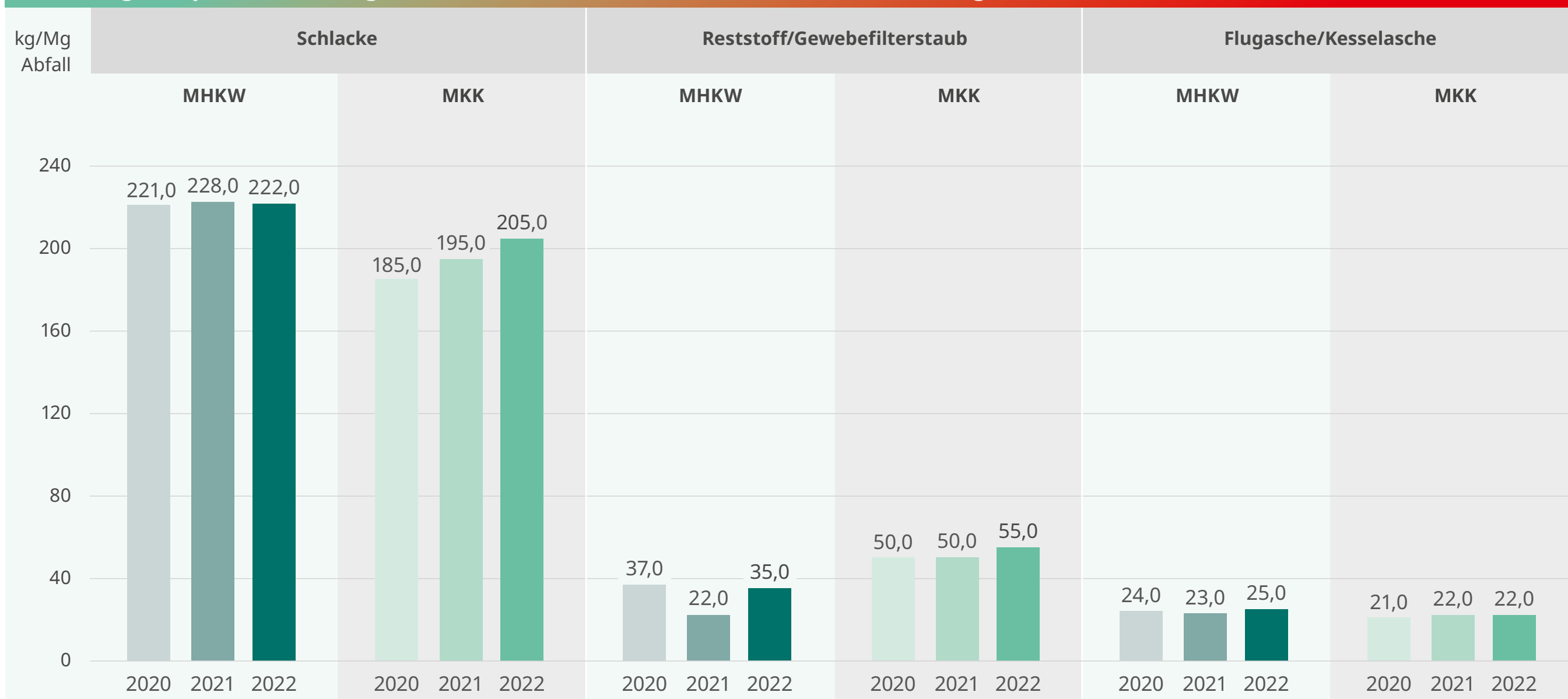
Abbildung 11 Spezifische Mengen Schlacke, Reststoff/Gewebefilterstaub sowie Flug- u. Kesselasche MHKW/MKK 2020–2022
